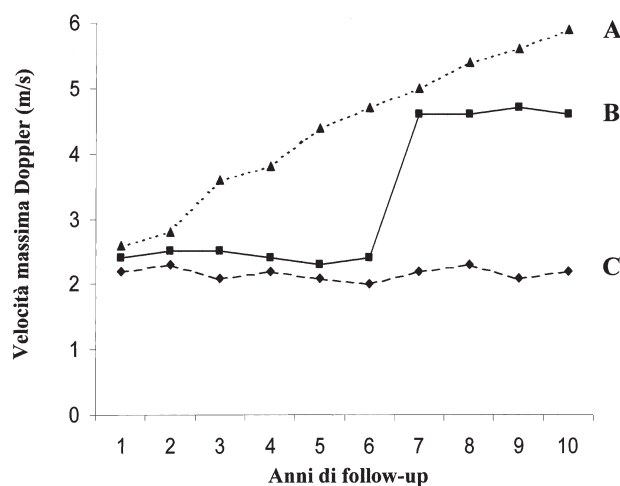
Figura 2. Modelli di progressione della stenosi aortica in 3 pazienti con stenosi aortica lieve seguiti con ecocardiogrammi seriali annuali per 10 anni. A: il paziente presenta un pattern di progressione lineare passando da una velocità del jet aortico iniziale di 2.6 m/s ad una finale di 5.9 m/s (tasso di incremento annuo di 0.33 m/s). B: il paziente presenta una progressione non lineare con gran parte dell'incremento di gradiente tra il sesto ed il settimo anno di follow-up. C: il paziente non modifica significativamente il grado di severità della stenosi aortica durante l'osservazione.
